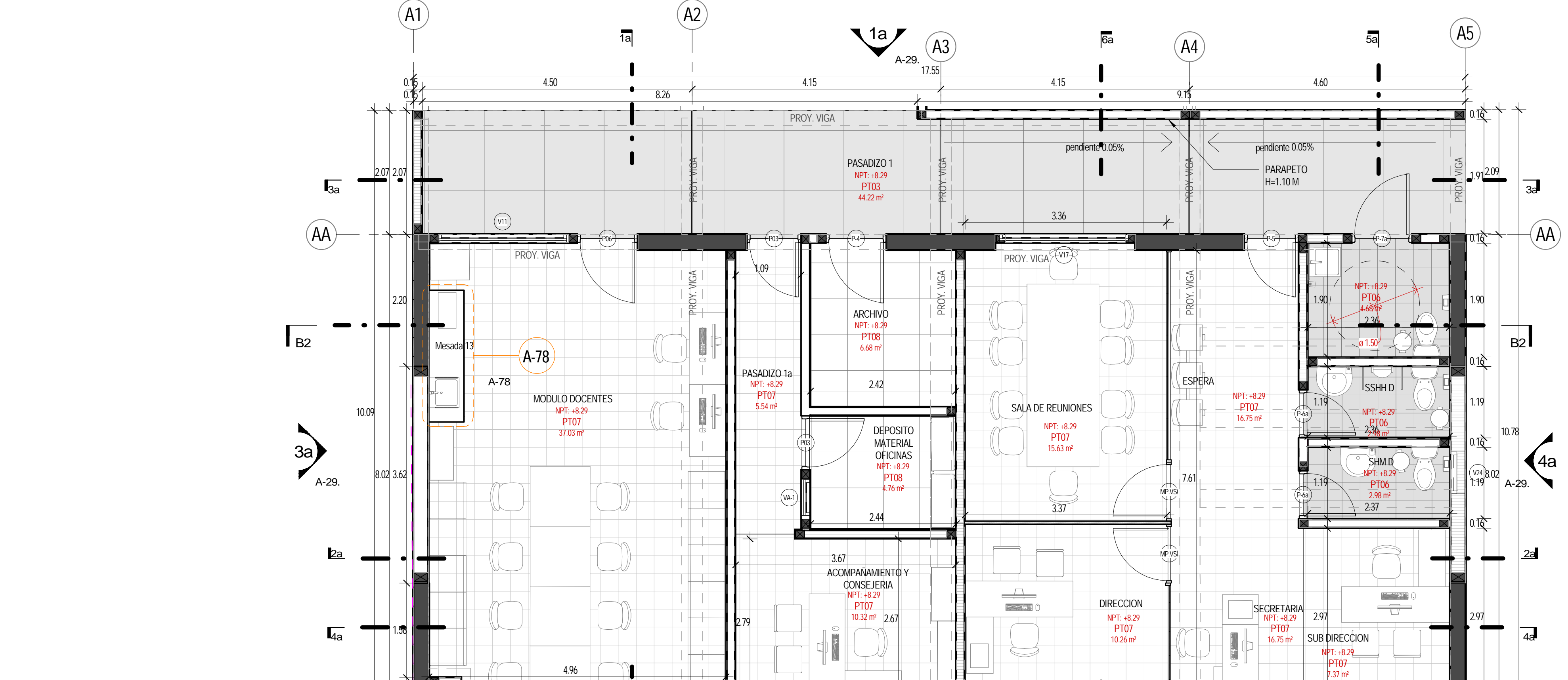
4 Nivel 8.07 piso 3 - Bloque A 1:50
