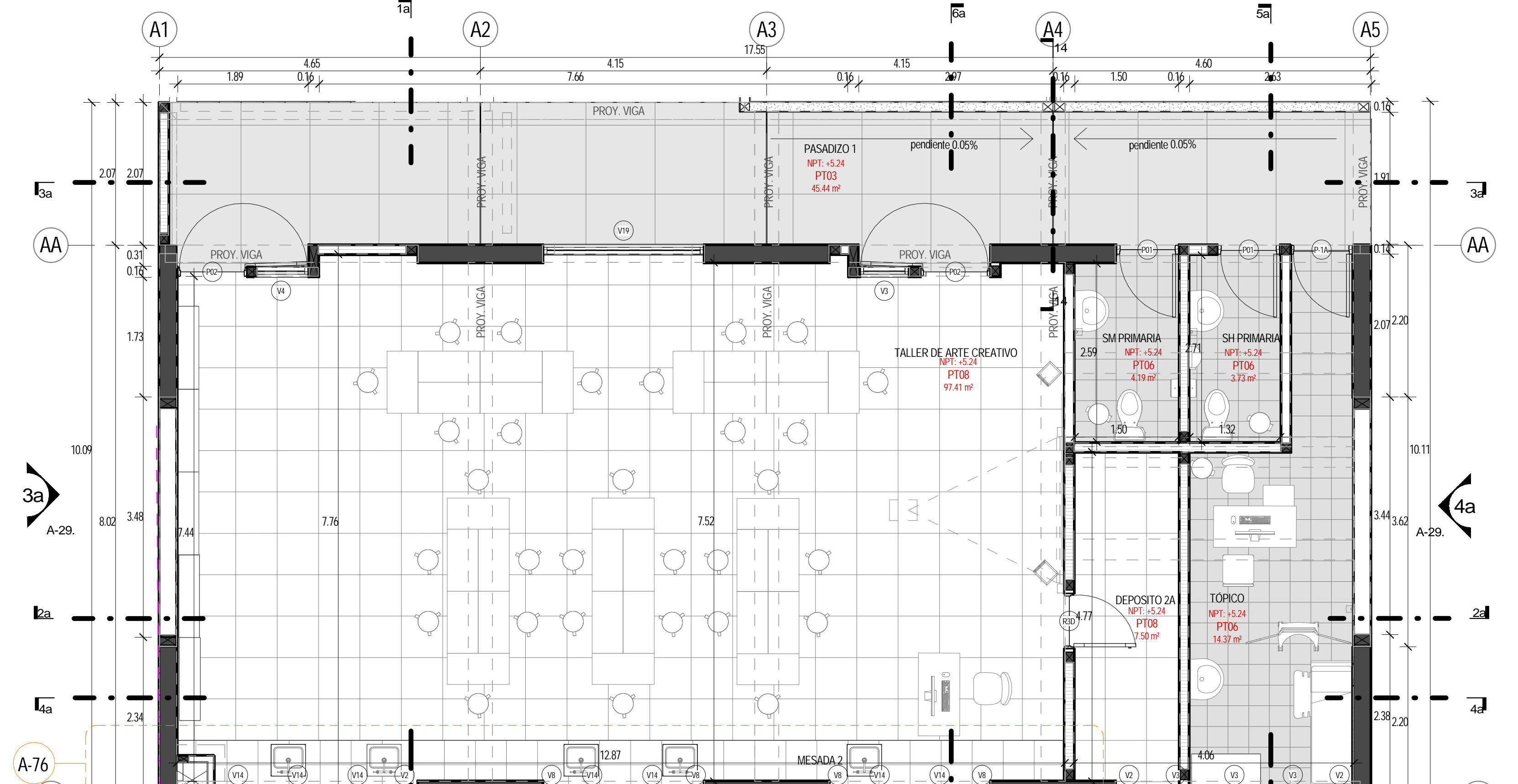
2 Nivel 5.02 piso 2 - Bloque A 1:50
